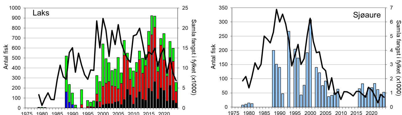
FIGUR 1. Fangst av laks og sjøaure i Espedalselva i perioden 1978–2024 (stolpar). Frå 1979 er laksefangstane skild som tert (<3 kg, grøn) og laks (>3 kg, blå), frå 1993 er det skild mellom smålaks (<3 kg, grøn), mellomlaks (3–7 kg, raud) og storlaks (>7 kg, svart). Linjer viser samla fangst av laks og sjøaure i resten av Rogaland (utanom Espedalselva). Sjøauren er freda frå 2010. NB! Figuren inkluderer gjenutsett fisk.
